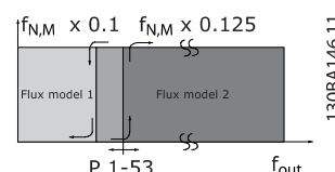
图 3.2: 参数 1-00 配置模式 = [1] 闭环速度或 [2] 转矩和 参数 1-01 电动机控制原理 = [3] 磁通矢量带电动机反馈
