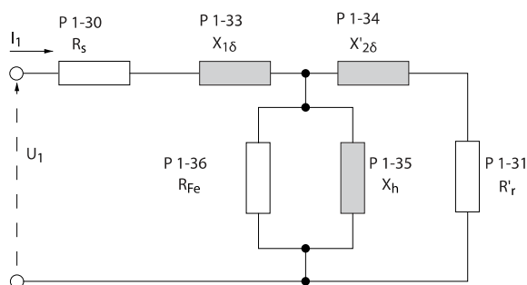
图 3.1: 异步电动机的电动机当量图
