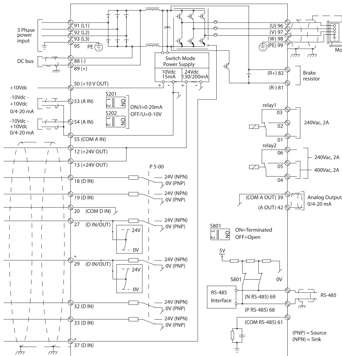
图 1.1: 图中显示了不带选件时的所有电气端子。
