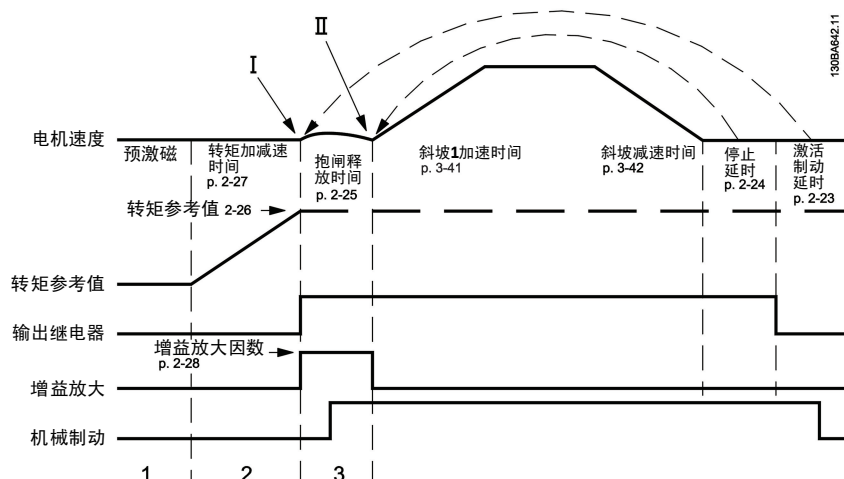
图 3.4: 起重机械制动控制的抱闸释放过程
