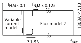
图 3.3: 参数 1-00 配置模式 = [0] 开环速度, 参数 1-01 电动控制原理 = [2] 无传感器矢量
