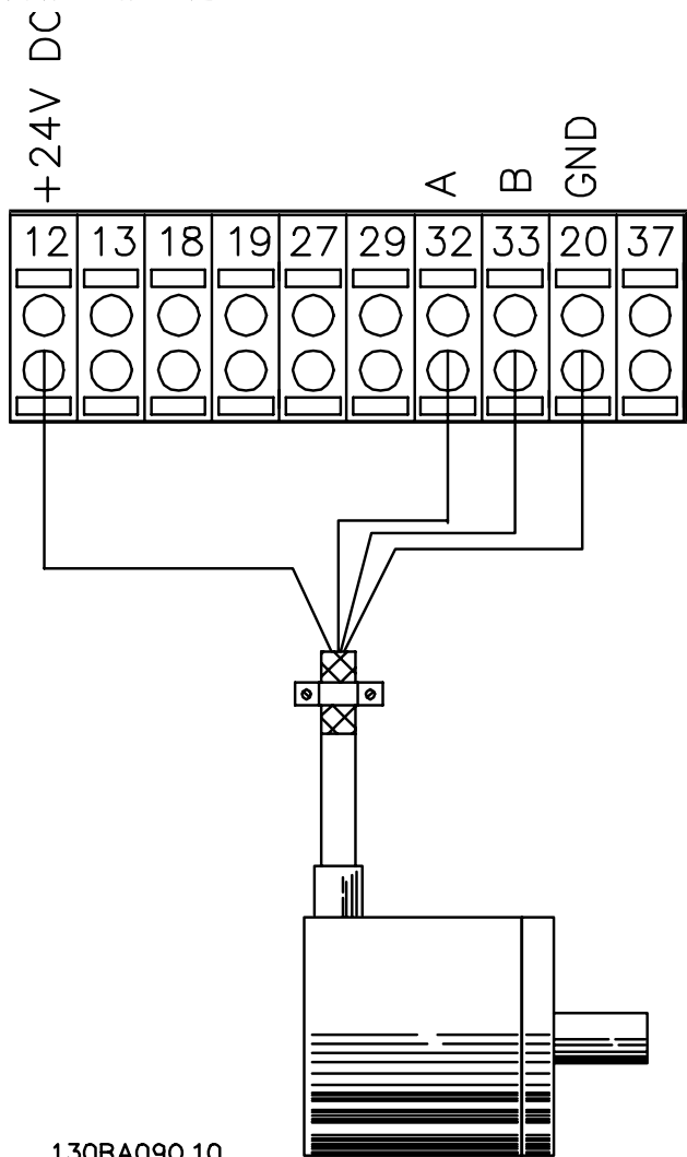
图 3.5: 24 V 增量编码器。电缆最大长度 5 m。
