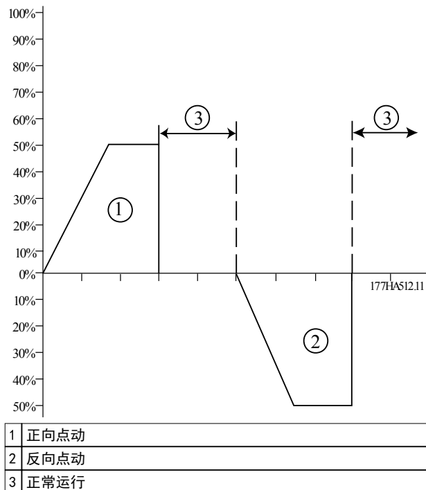
图 5.9 点动操作
