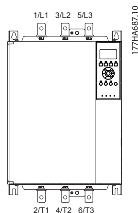
图 4.4 MCD5-0131B 至 MCD5-0215B, 131 - 215 A
