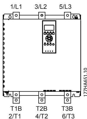
图 4.7 MCD5-0245C 上的旁路端子, 245 A
