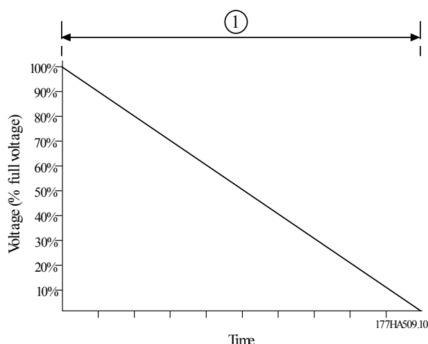
图 5.6 TVR 软停止
