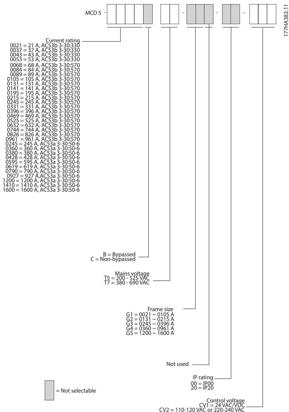
图 1.1 类型代码订购表
