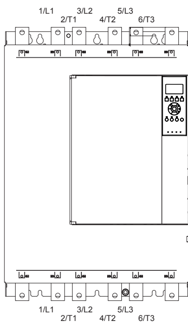
图 4.6 MCD5-0469B 至 MCD5-0961B, 469 - 961 A
