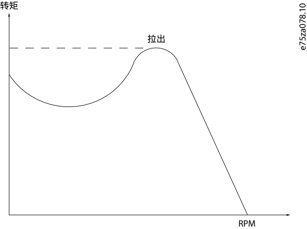
图 22: 起步转矩
