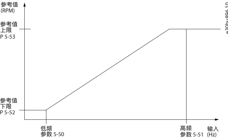
图 14: 脉冲输入
