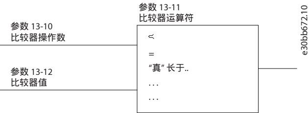
图 16: 比较器
