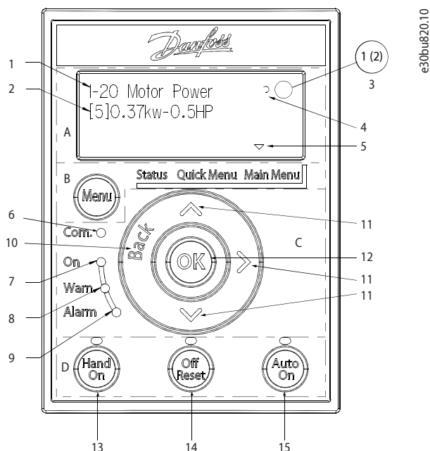
图 2: 本地控制面板 (LCP 32)
