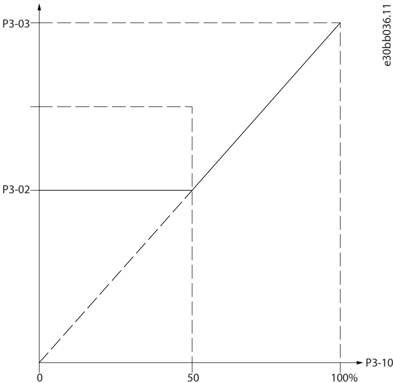
图 9: 参考值
