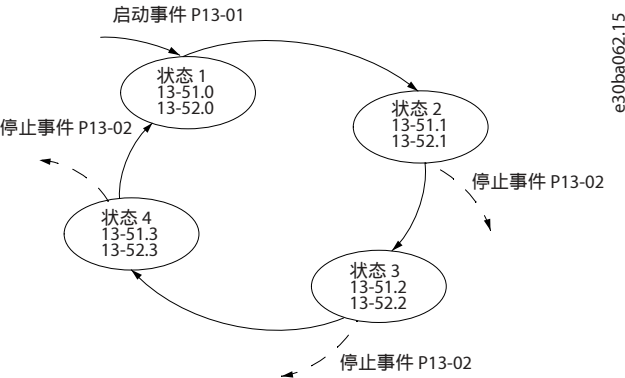
图 15: 3 个事件/操作示例
