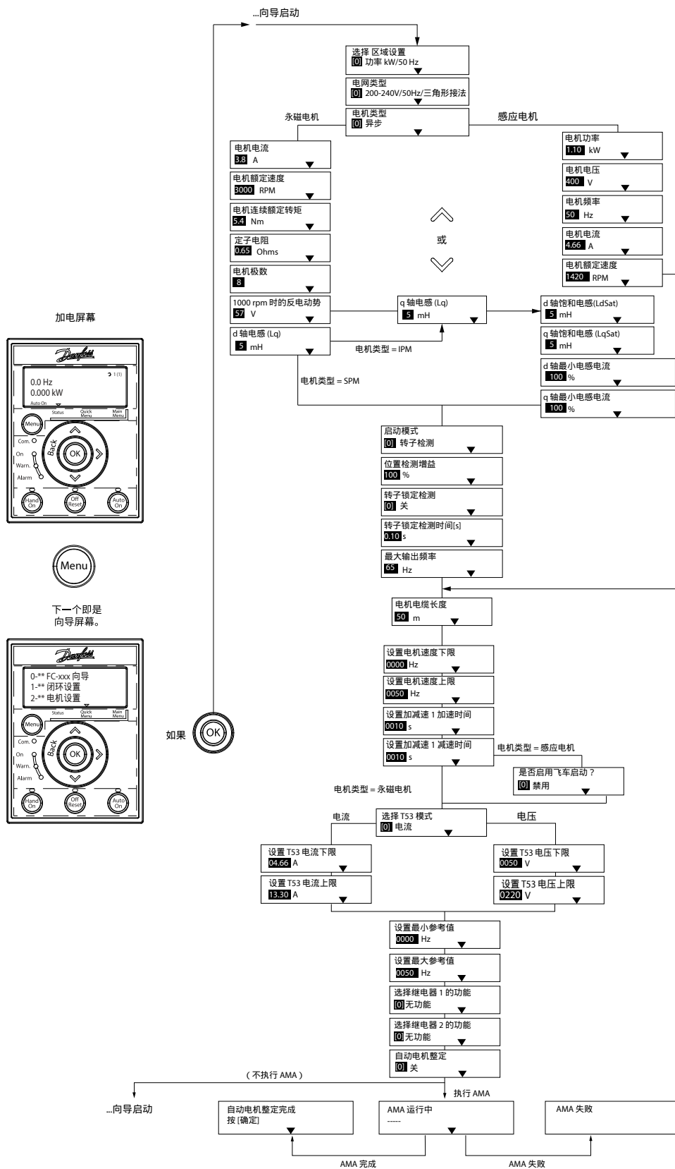
图 4: 开环应用设置向导
