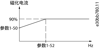
图 7: 电机磁化
