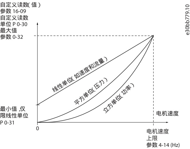
图 6: 自定义读数
