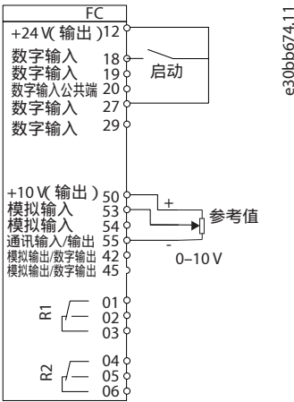
图 3: 变频器接线
