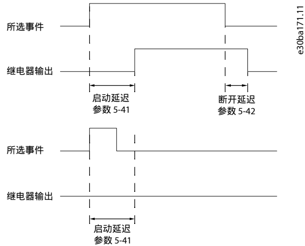
图 12: 继电器打开延迟
