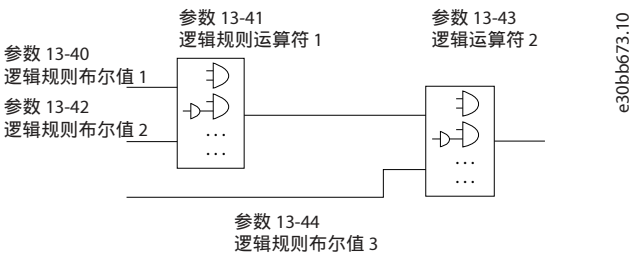
图 17: 逻辑规则
