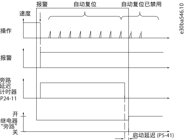
图 20: 变频器旁路
