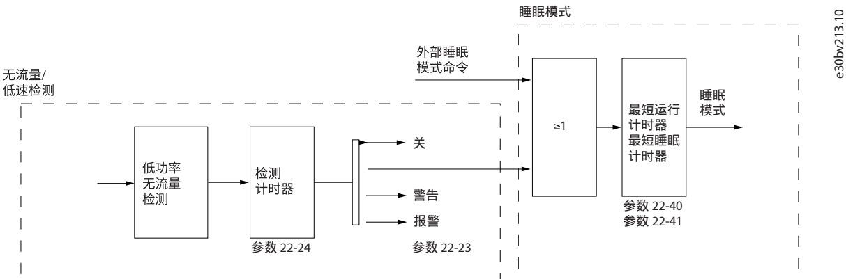
图 18: 无流量检测
