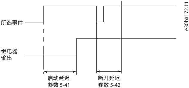
图 13: 继电器打开延迟
