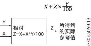
图 10: 预置相对参考值
