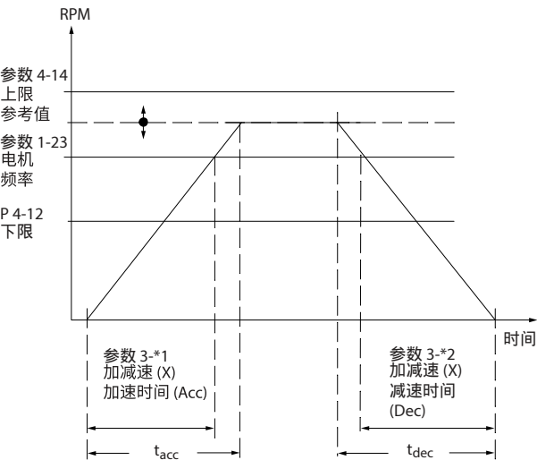
图 11: 加减速
