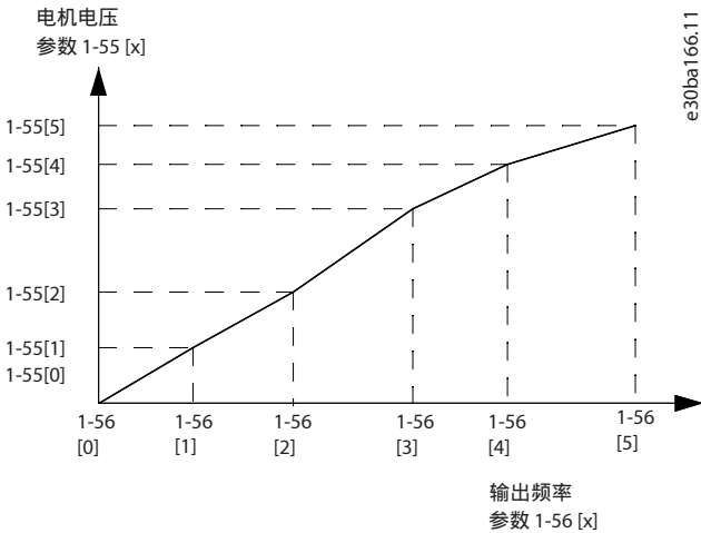
图 8: U/f 特性
